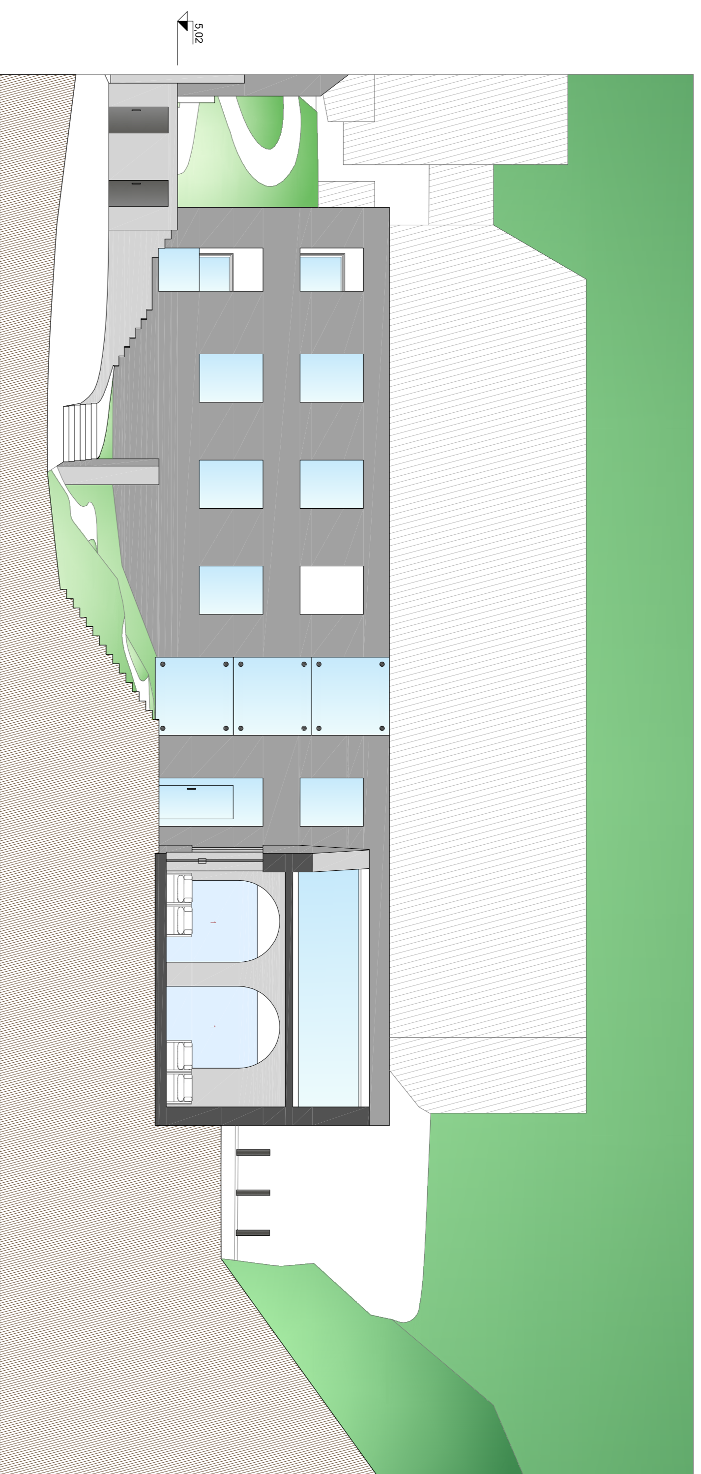
CORTE 88 Esc. 1/100
