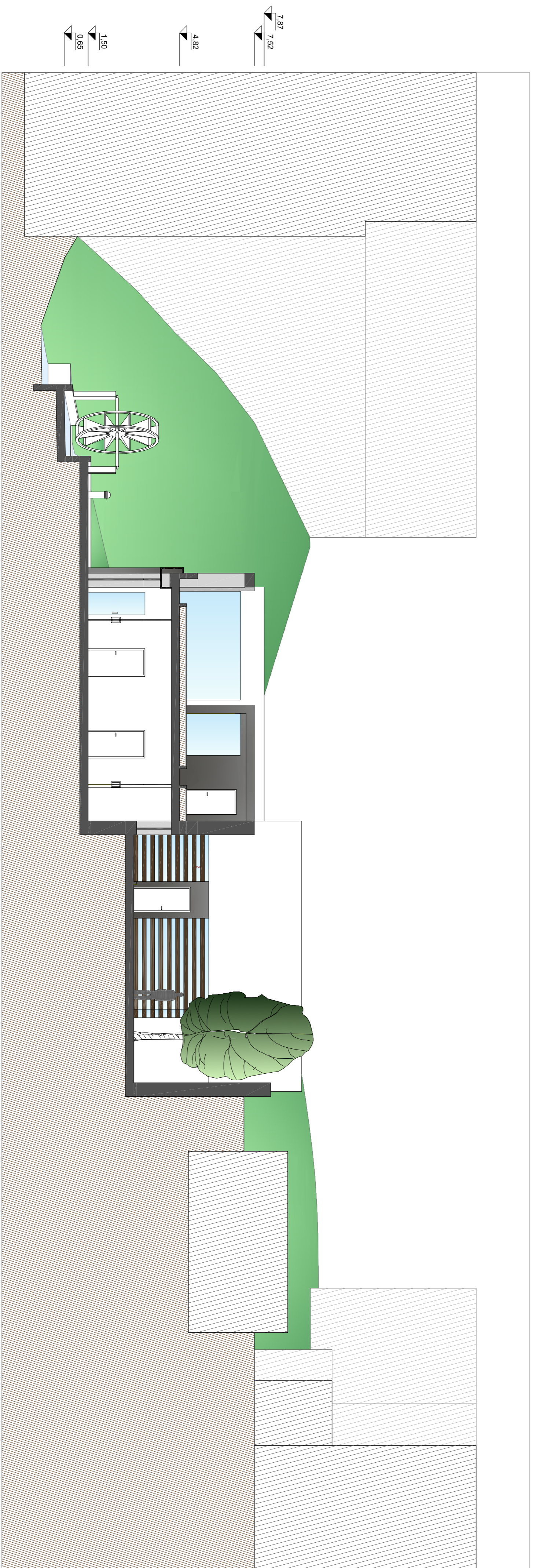
CORTE 89 Esc. 1/100
