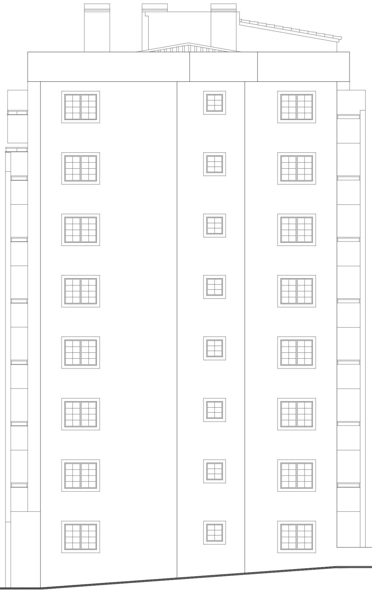
ALÇADO NORTE
