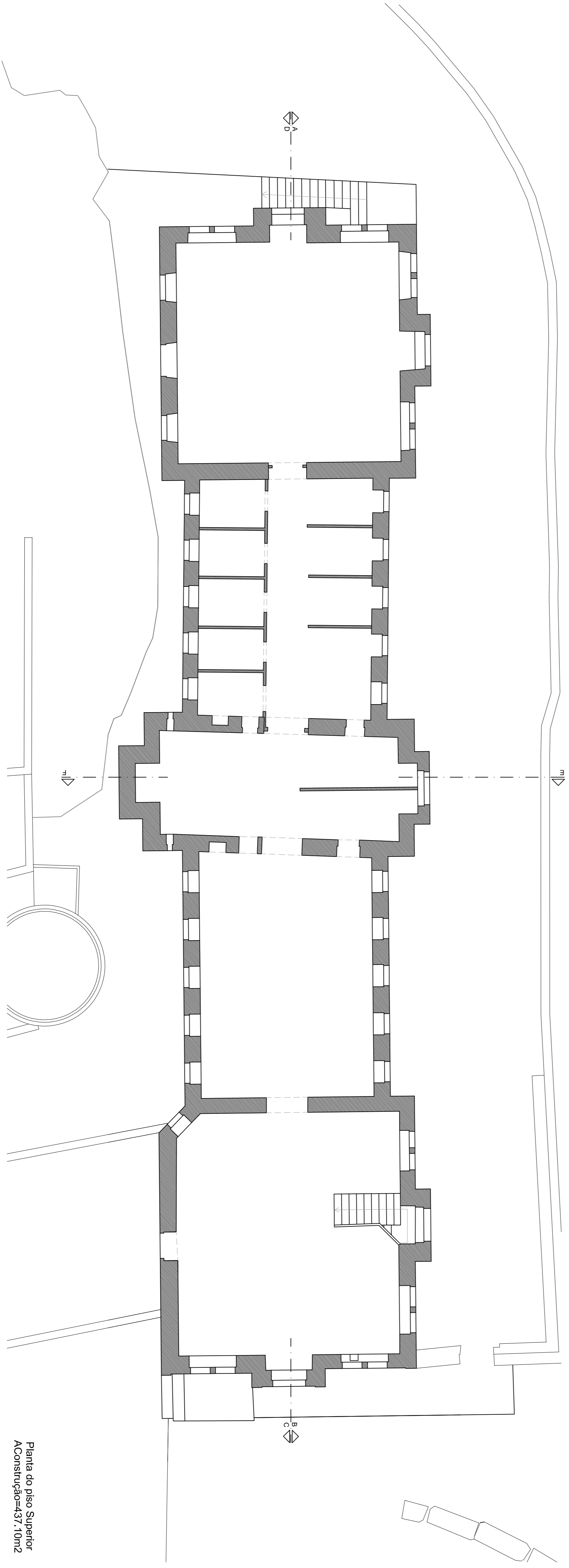
Planta do piso Inferior AConstrução=312,50m 2
