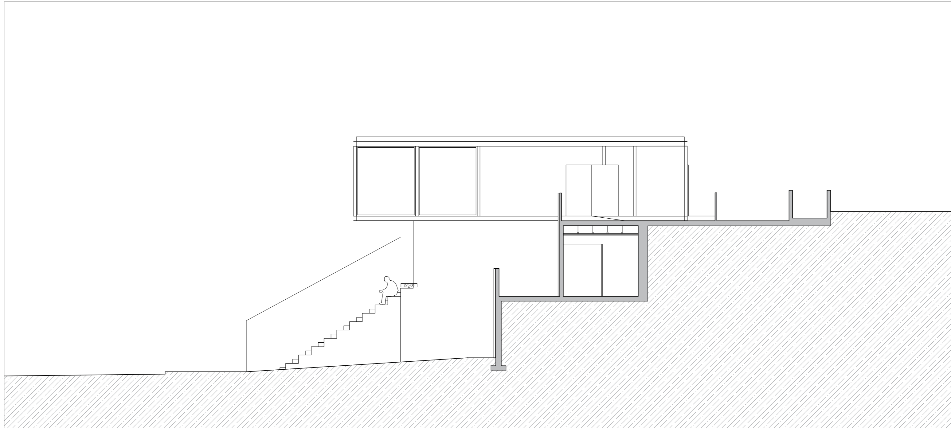
CORTE E2 ANEXOS CASA PINA FALCÃO
